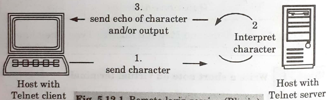
Fig. 5.12.1. Remote login session (Rlogin).
