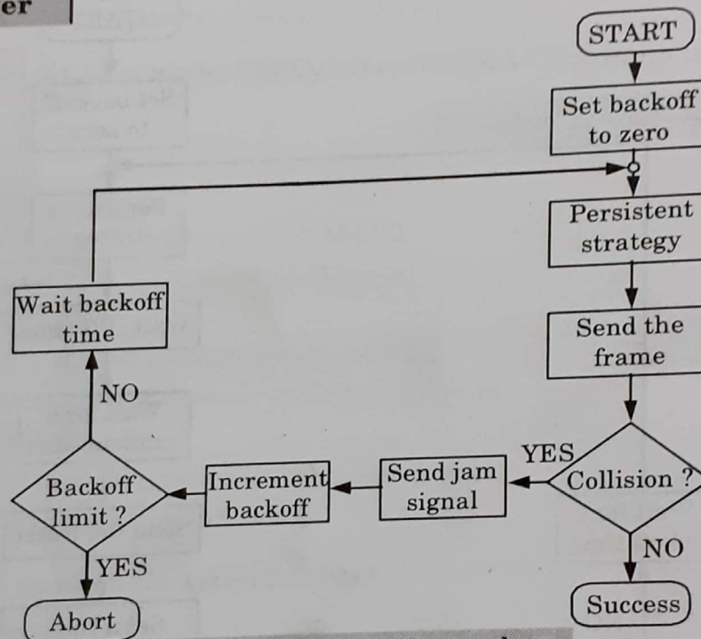
Fig. 2.5.1. CSMA/CD procedure.
