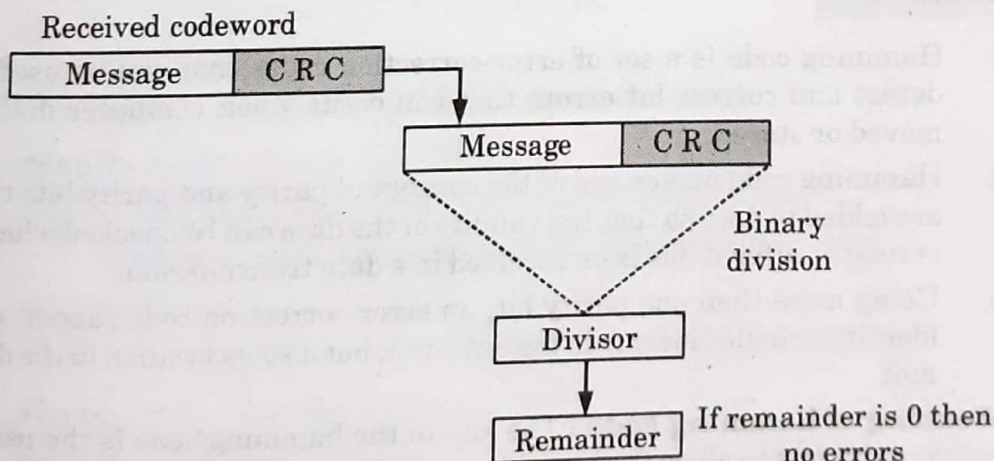
Fig. 2.34.2. CRC checker.
