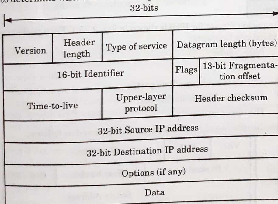
Fig. 3.22.1. IPv4 datagram format.
