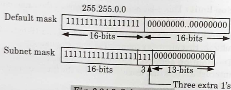
Fig. 3.24.2. Subnet mask.
