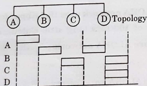
Fig. 2.10.1. Slotted ALOHA.
