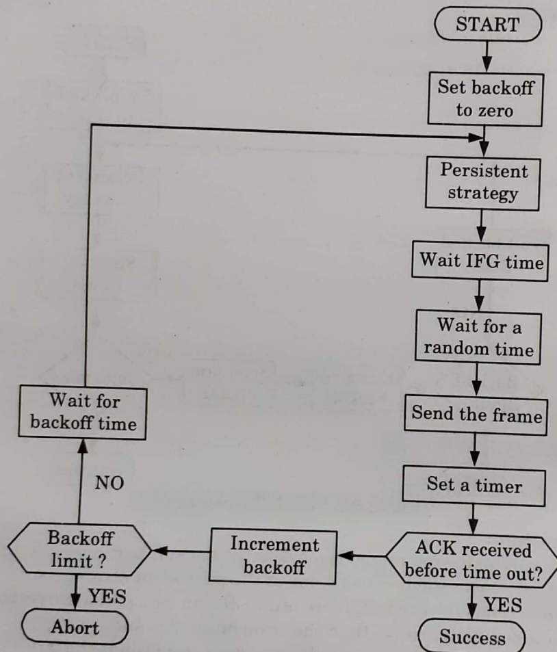
Fig. 2.6.1. CSMA / CA procedure.
