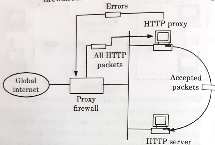
Fig. 5.12.4. Proxy firewall.
