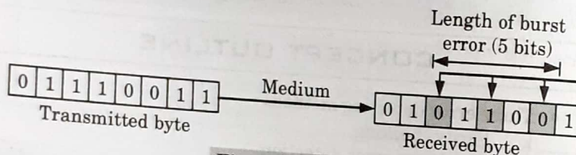
Fig. 2.31.2. Burst error.
