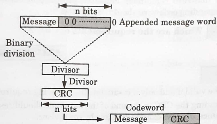
Fig. 2.34.1. CRC generator.
