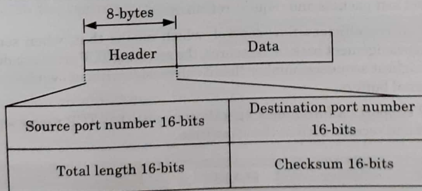
Fig. 4.5.1. User datagram format.
